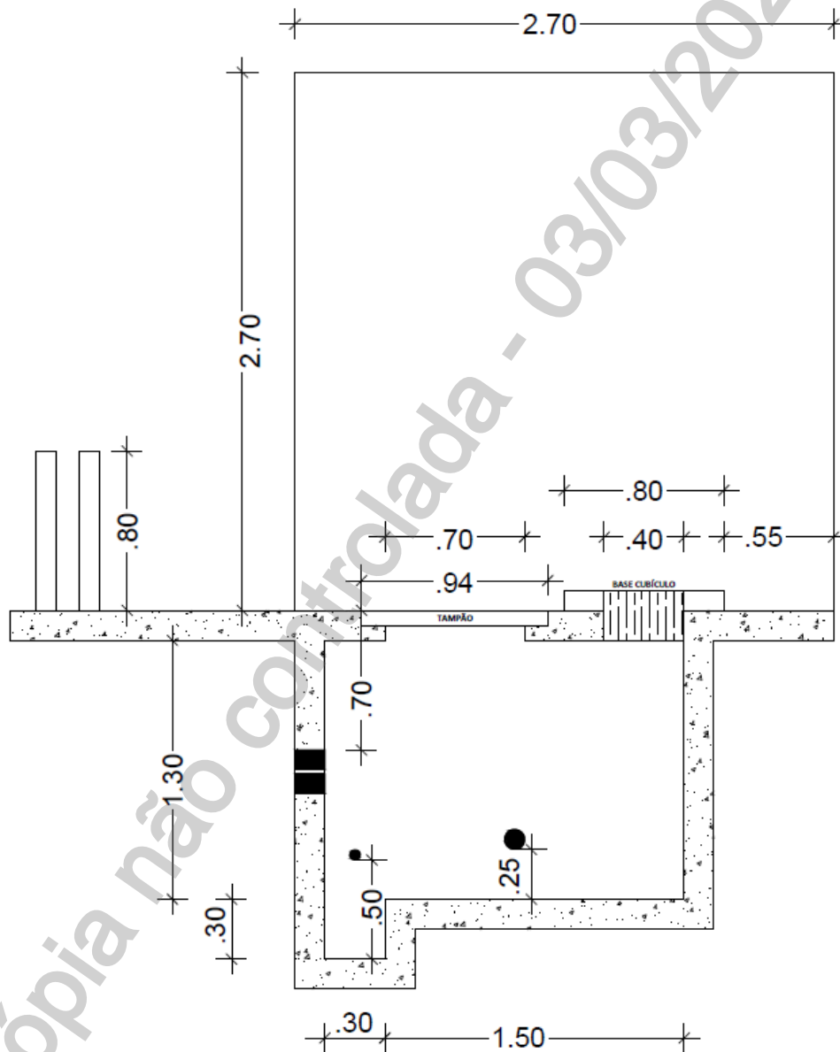
Desenho 8 - CTE para 1 Transformador de até 225 kVA - 4/9 (CTE-R-225/CTE-225-RE+P/ CTE-225-RE+2P/ CTE-225-RE+3P)
