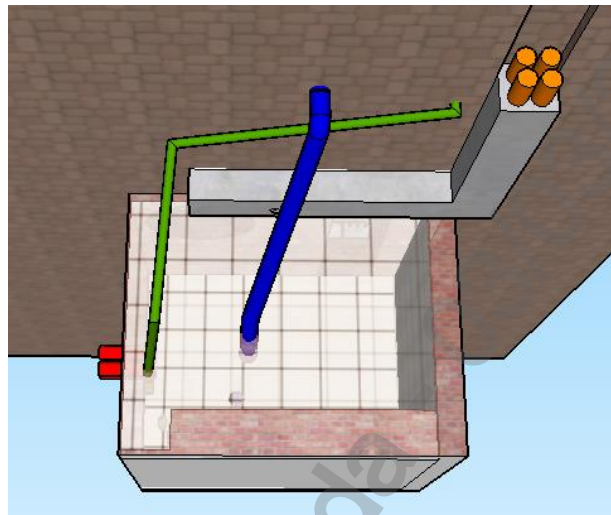
Desenho 9 - CTE para 2 Transformadores de até 225 kVA - 10/10 (CTE-R-450-RE+2P/ CTE-R-450-RE+3P/CTE-A-2L+P)
