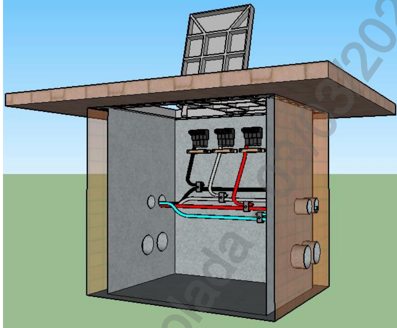
Desenho 18 - Poço Primário (PP) - 15 kV - 5/6
