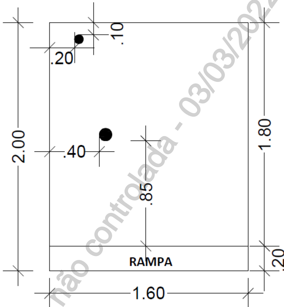
Desenho 1 – Base do Transformador de 15 kV – 1/4
