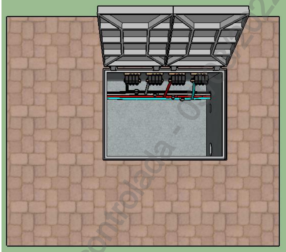
Desenho 19 - Poço Primário (PE) - 15 kV - 4/7
