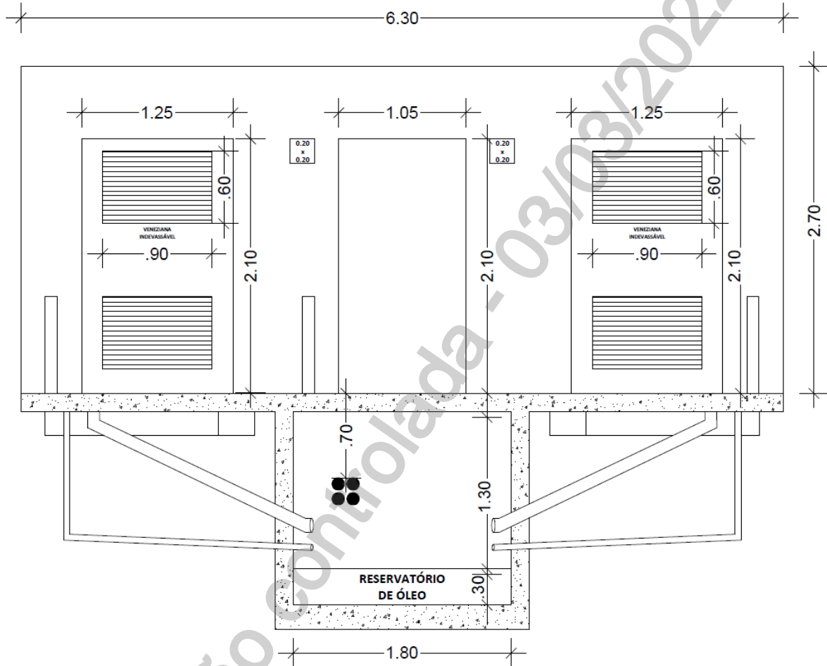
Desenho 11 - CTE para 2 Transformadores de até 225 kVA - 2/8 (CTE-R-450-RE+2P/ CTE-R-450-RE+3P/CTE-A-2L+P)
