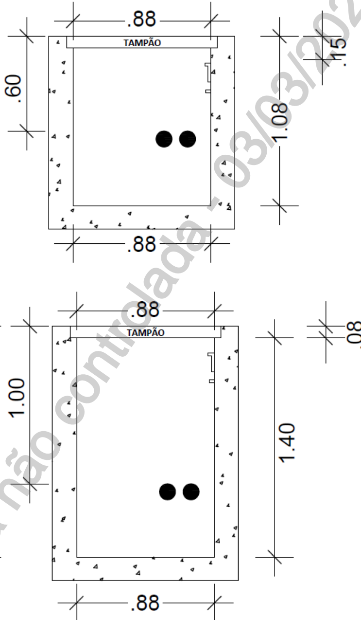
Desenho 15 - Poço Secundário (PS1) - 4/7
