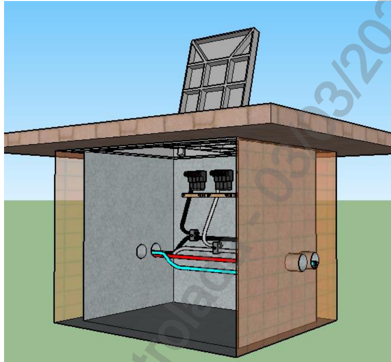
Desenho 15 - Poço Secundário (PS1) - 6/7
