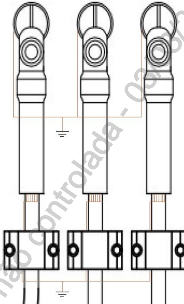
Desenho 48 – Aterramento dos Cabos na Estrutura Interna da CTE/CM com Uso de Desconectável
