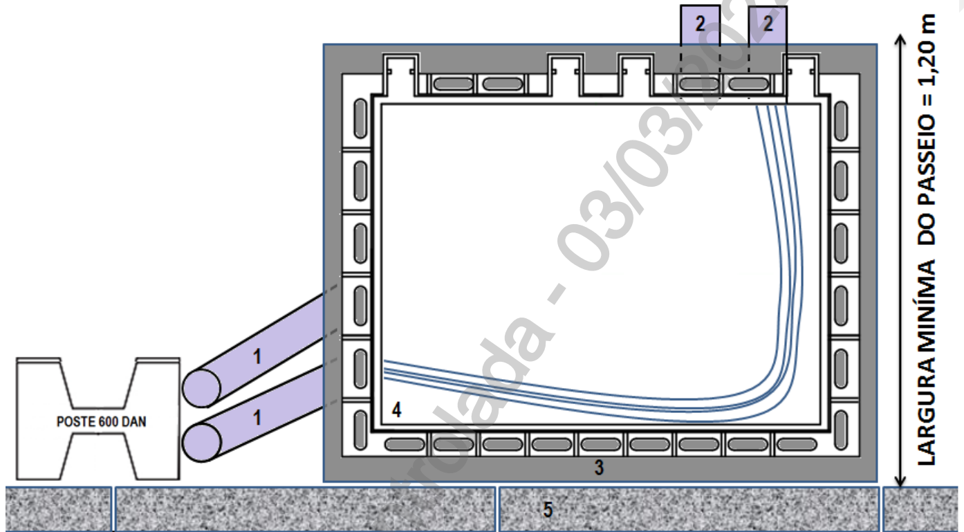
Desenho 26 - Representação Descida do Poste com Poço PS1 para Rede de BT
