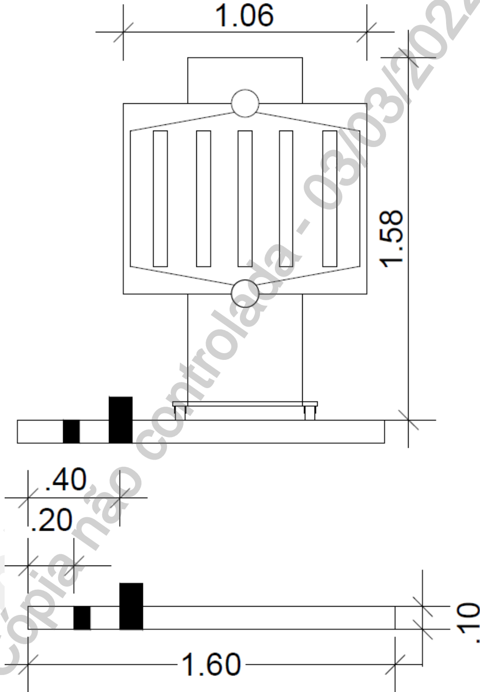
Desenho 1 – Base do Transformador de 15 kV – 3/4
