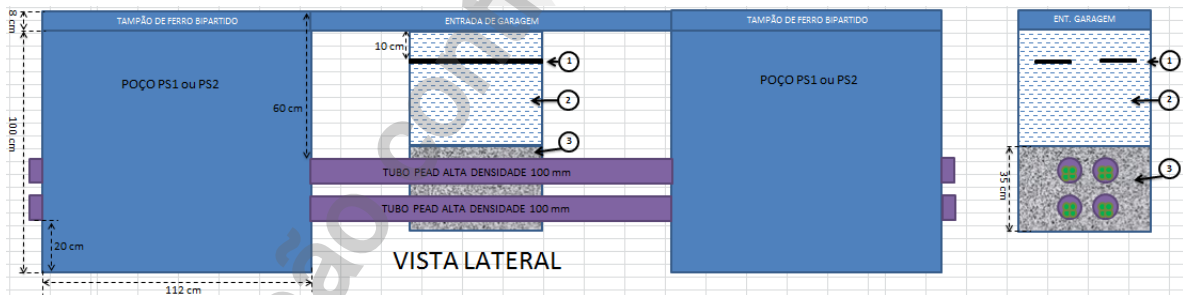
Eletrودuto de polietileno de alta densidade (PEAD) em entrada de garagem
