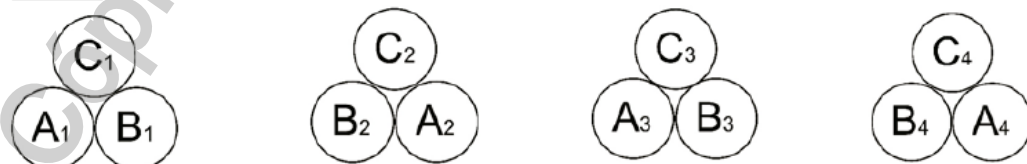
Figura 2 – Transposição das Fases dos Cabos em Bandeja ou Calha (Trifólio)
