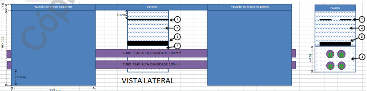
Eletrودuto de polietileno de alta densidade (PEAD) em passeio
