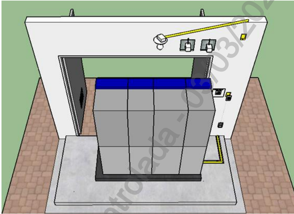
Desenho 14 - CM-R-RE+2P/ CM-R-RE+3P/CM-A-3L/ CM-A-4L Câmara de Manobra – 7/7
