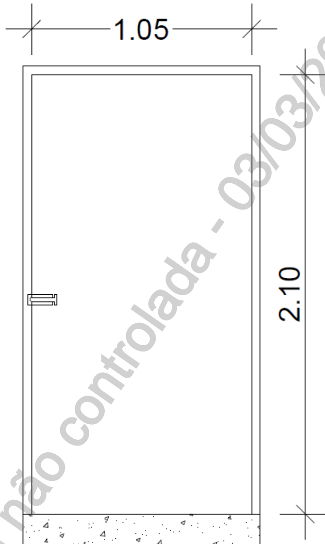
Desenho 3 - Portas de Acesso de Pessoas em Câmara de Transformação
