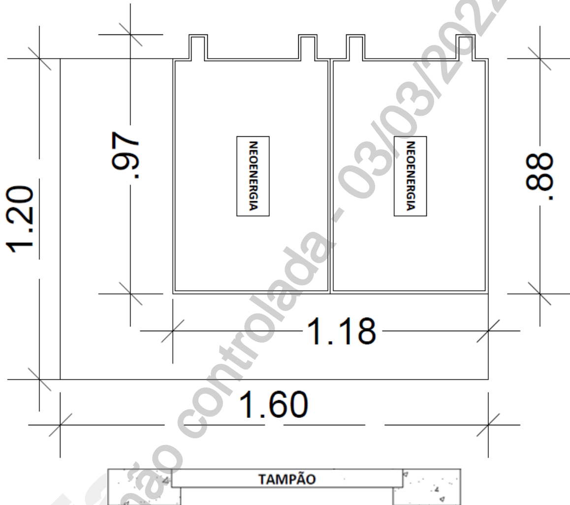
Desenho 19 - Poço Primário (PE) - 15 kV - 1/7
