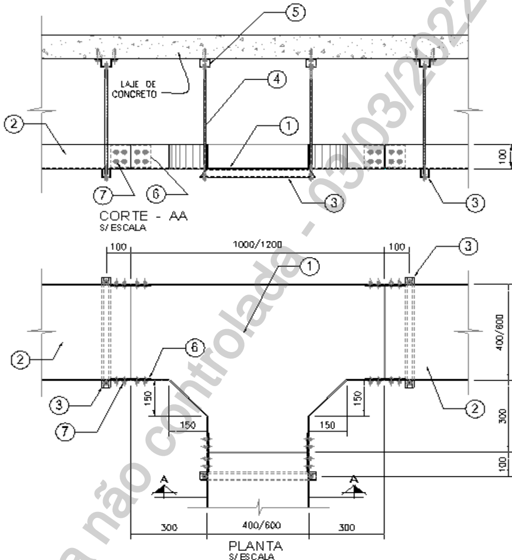
DETALHE - 2 BANDEJA - JUNÇÃO EM TÊ RETO 90°
