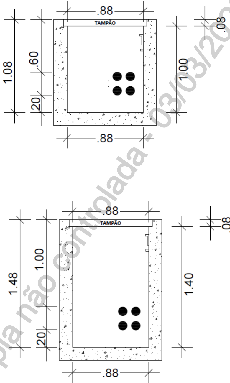
Desenho 16 - Poço Secundário (PS2) - 4/4
