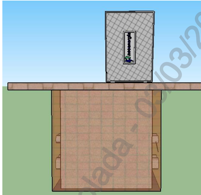
Desenho 18 - Poço Primário (PP) - 15 kV - 6/6
