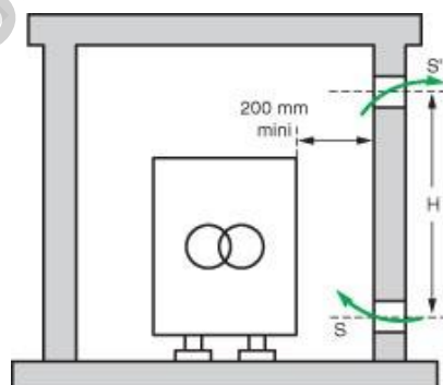
Figura 4 - Troca de Calor pelo Modo de Convecção Livre
