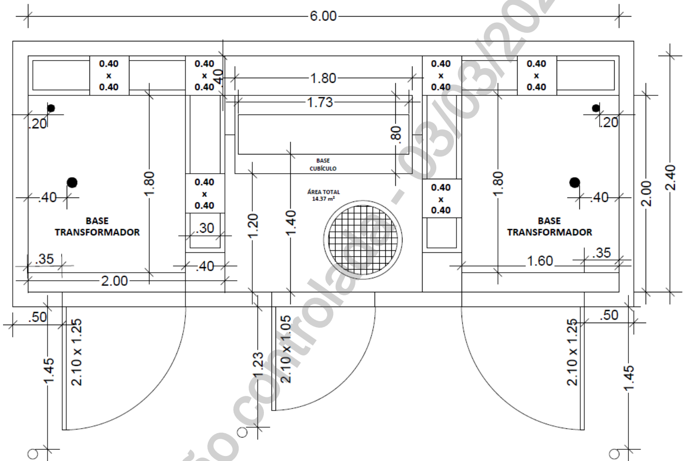
Desenho 9 - CTE para 2 Transformadores de até 225 kVA - 1/10 (CTE-R-450-RE+2P/ CTE-R-450-RE+3P/CTE-A-2L+P)
