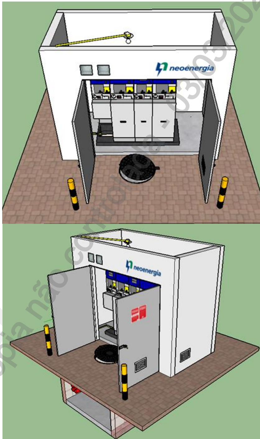
Desenho 14 - Câmara de Manobra - 6/7 (CM-R-RE+2P/ CM-R-RE+3P/CM-A-3L/ CM-A-4L)
