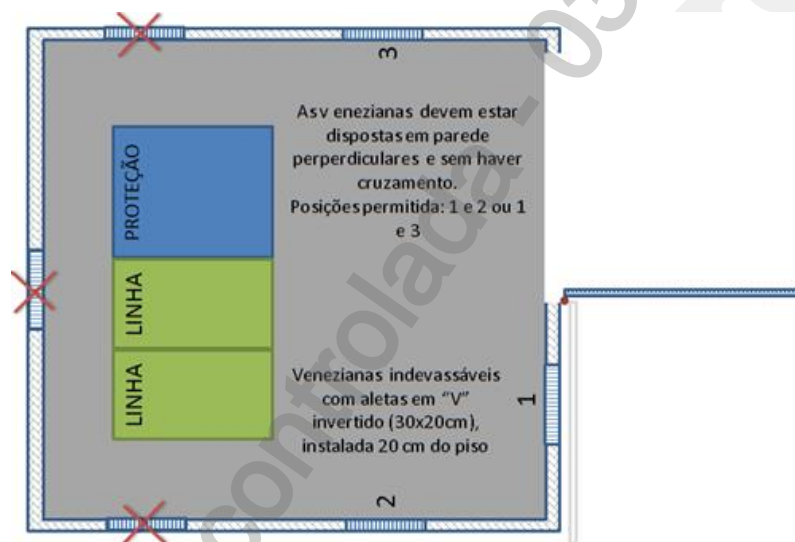
Figura 8 - Posição das Venezianas
