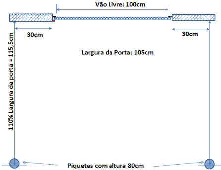
Figura 9 - Representação dos Vãos Livres das Portas em Função da Aplicação
