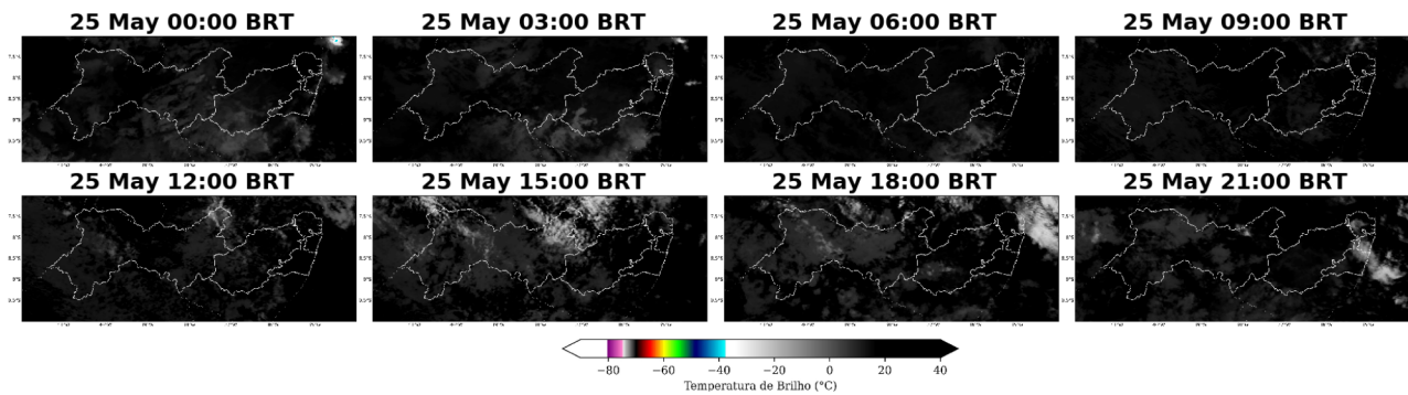
Figura 8: Imagens realçadas do satélite GOES-16 das 00 BRT até 21 BRT (a cada 3 horas) para o dia 25 de maio.
