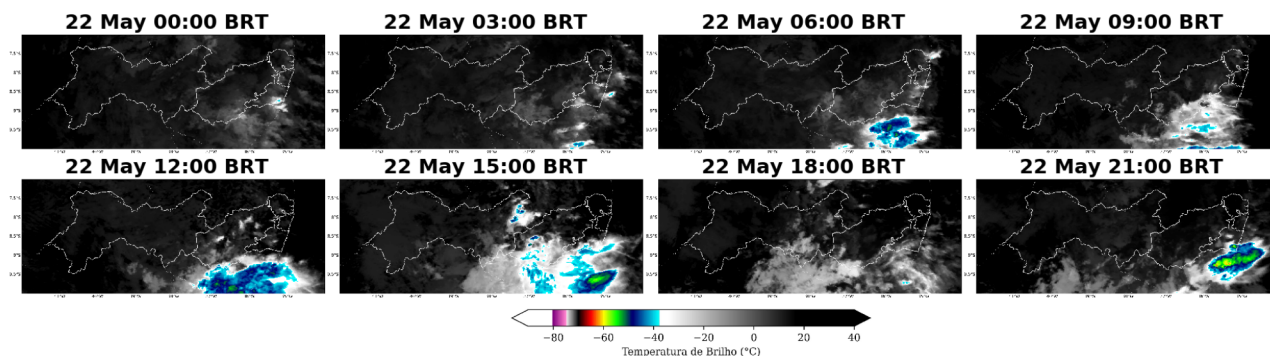
Figura 5: Imagens realçadas do satélite GOES-16 das 00 BRT até 21 BRT (a cada 3 horas) para o dia 22 de maio.
