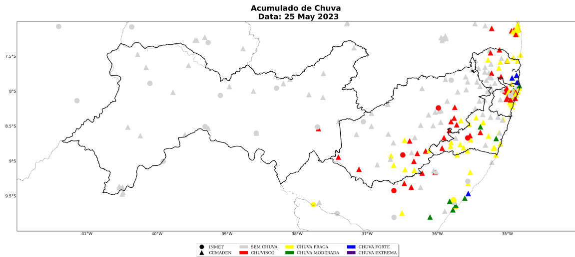
Figura 15: Acumulado diário de precipitação sobre o estado de Pernambuco para o dia 25 de maio, baseado nas estações meteorológicas do INMET e CEMADEN
