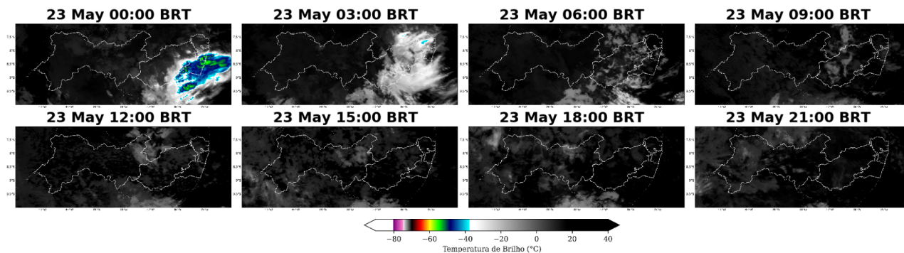
Figura 6: Imagens realçadas do satélite GOES-16 das 00 BRT até 21 BRT (a cada 3 horas) para o dia 23 de maio.
