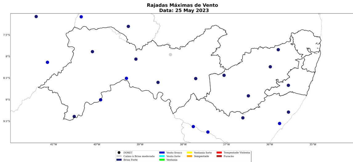
Figura 25: Rajada de vento sobre o estado de Pernambuco para o dia 25 de maio, baseado nas estações meteorológicas do INMET
