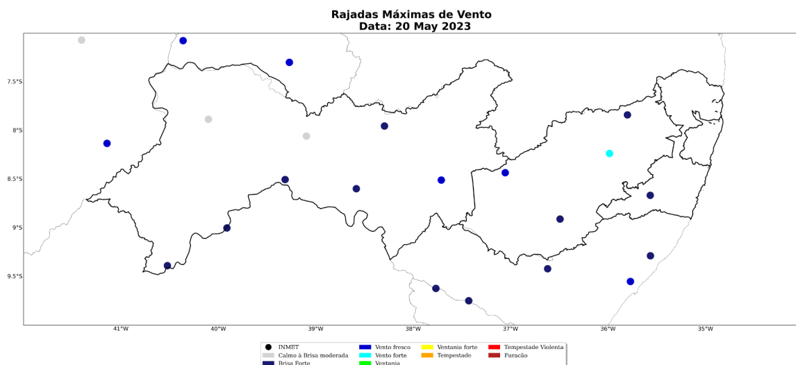
Figura 20: Rajada de vento sobre o estado de Pernambuco para o dia 20 de maio, baseado nas estações meteorológicas do INMET
