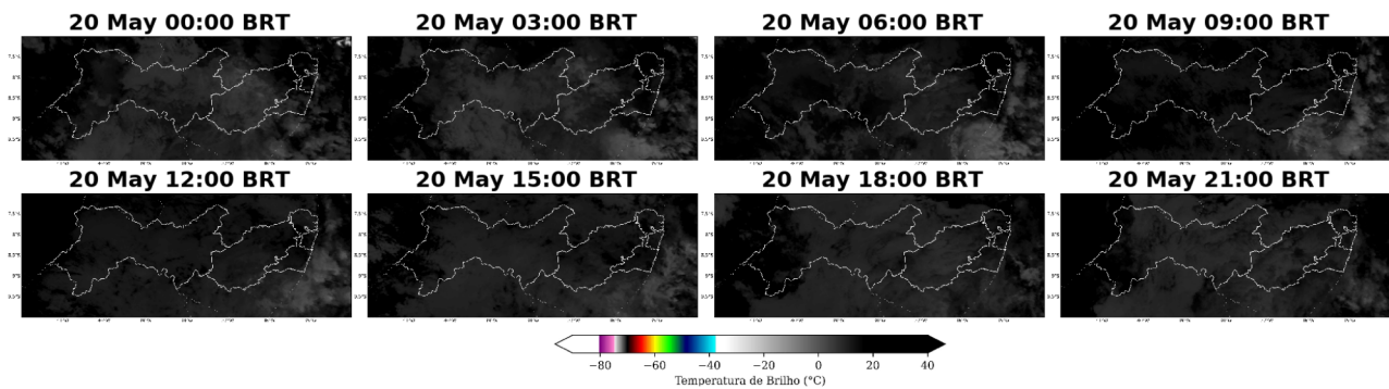
Figura 3: Imagens realçadas do satélite GOES-16 das 00 BRT até 21 BRT (a cada 3 horas) para o dia 20 de maio.
