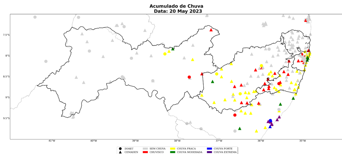
Figura 10: Acumulado diário de precipitação sobre o estado de Pernambuco para o dia 20 de maio, baseado nas estações meteorológicas do INMET e CEMADEN
