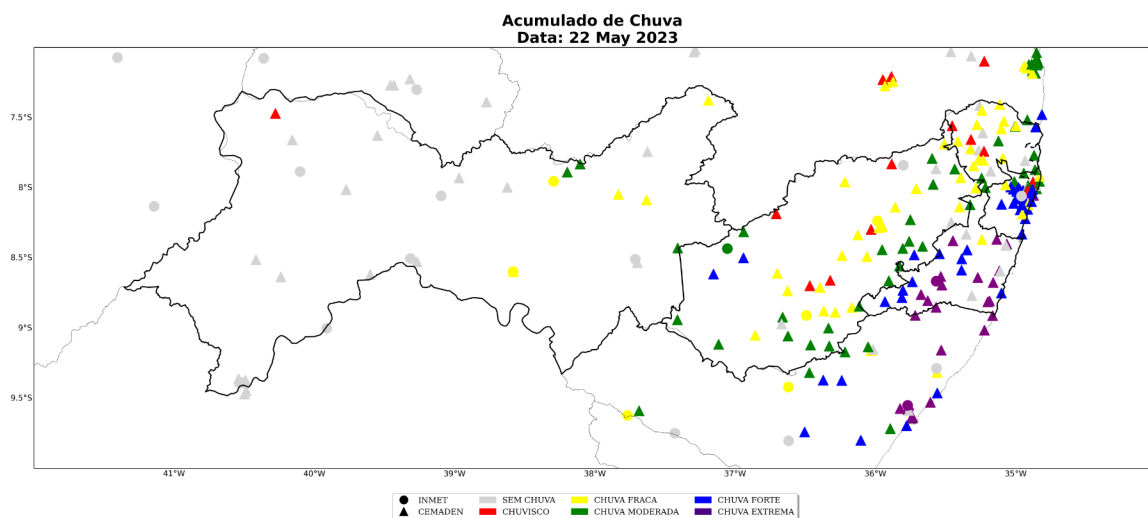
Figura 12: Acumulado diário de precipitação sobre o estado de Pernambuco para o dia 22 de maio, baseado nas estações meteorológicas do INMET e CEMADEN
