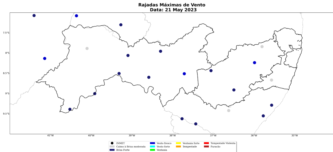
Figura 21: Rajada de vento sobre o estado de Pernambuco para o dia 21 de maio, baseado nas estações meteorológicas do INMET
