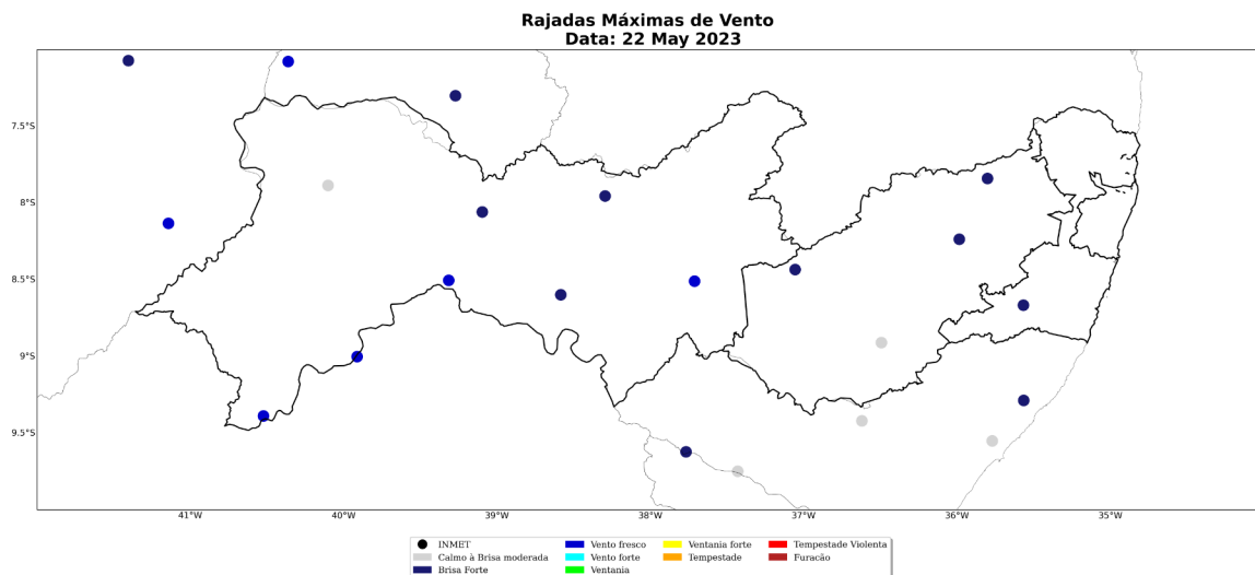
Figura 22: Rajada de vento sobre o estado de Pernambuco para o dia 22 de maio, baseado nas estações meteorológicas do INMET
