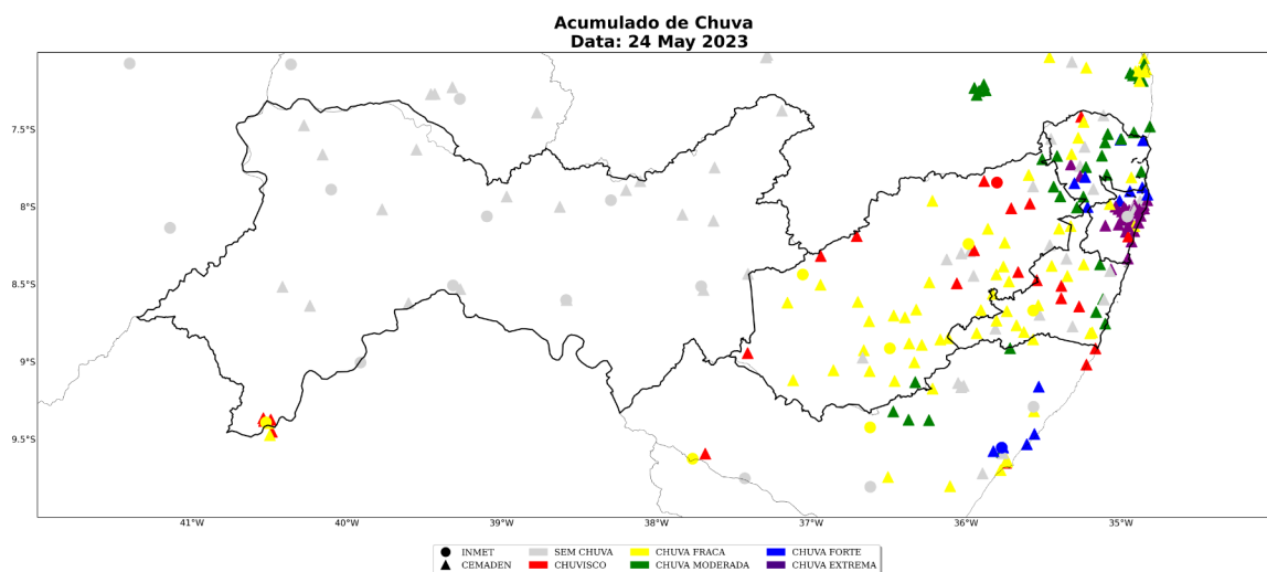
Figura 14: Acumulado diário de precipitação sobre o estado de Pernambuco para o dia 24 de maio, baseado nas estações meteorológicas do INMET e CEMADEN
