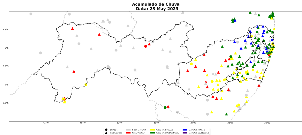
Figura 13: Acumulado diário de precipitação sobre o estado de Pernambuco para o dia 23 de maio, baseado nas estações meteorológicas do INMET e CEMADEN
