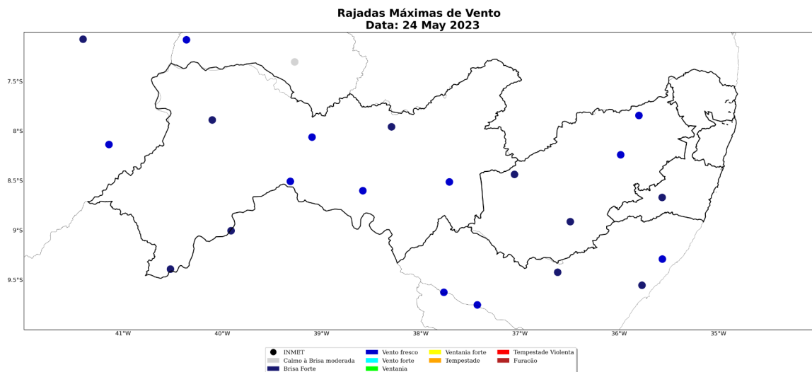
Figura 24: Rajada de vento sobre o estado de Pernambuco para o dia 24 de maio, baseado nas estações meteorológicas do INMET
