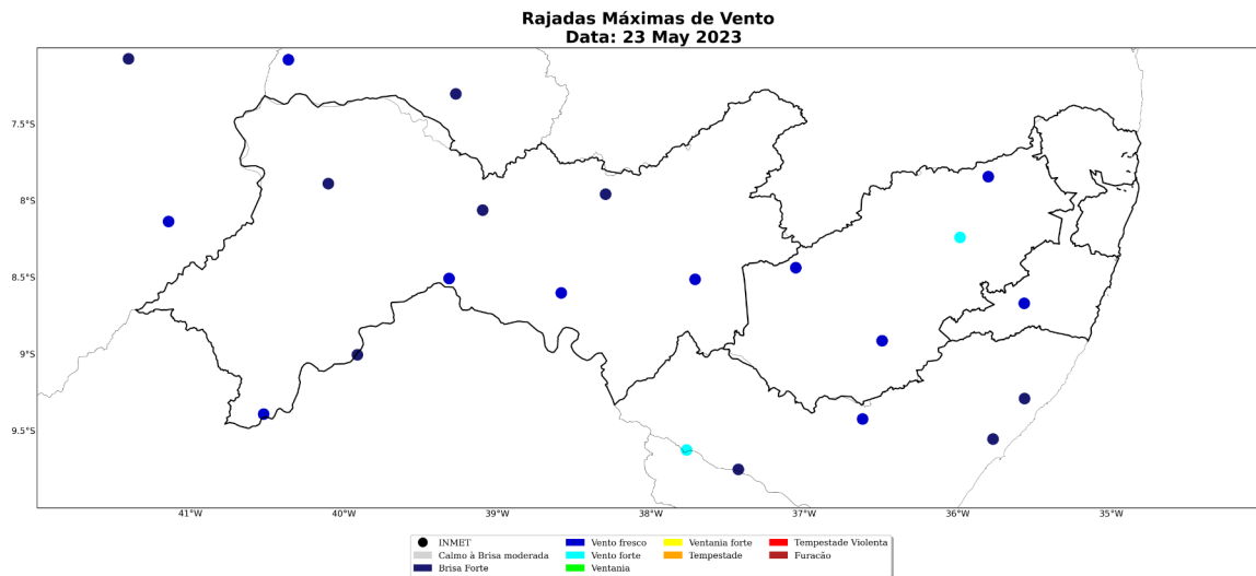
Figura 23: Rajada de vento sobre o estado de Pernambuco para o dia 23 de maio, baseado nas estações meteorológicas do INMET
