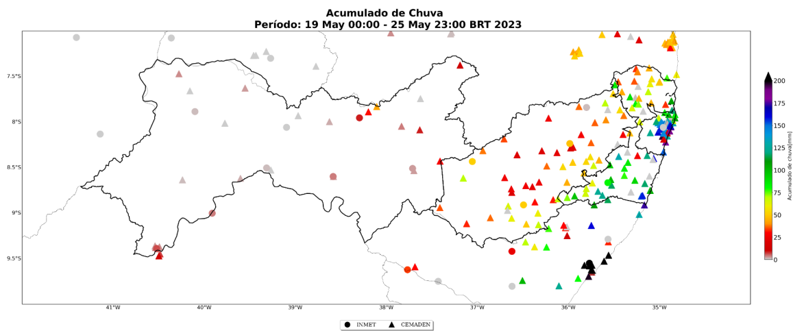
Figura 16: Acumulado de precipitação sobre o estado do Pernambuco para o período do evento (dias 19 a 25 de maio de 2023), baseado nas estações meteorológicas do INMET e CEMADEN.
