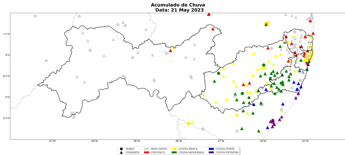
Figura 11: Acumulado diário de precipitação sobre o estado de Pernambuco para o dia 21 de maio, baseado nas estações meteorológicas do INMET e CEMADEN
