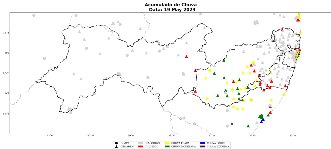
Figura 9: Acumulado diário de precipitação sobre o estado de Pernambuco para o dia 19 de maio, baseado nas estações meteorológicas do INMET e CEMADEN
