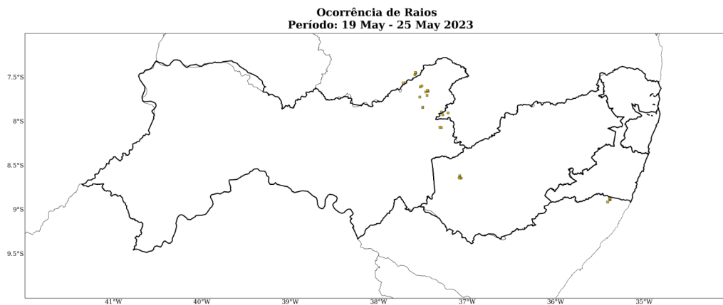
Figura 18: Ocorrência de descargas atmosféricas nuvem-solo detectadas pelo sistema Earth Networks para o período de 19 a 25 de maio de 2023 sobre a área de concessão da Neoenergia - Pernambuco.
