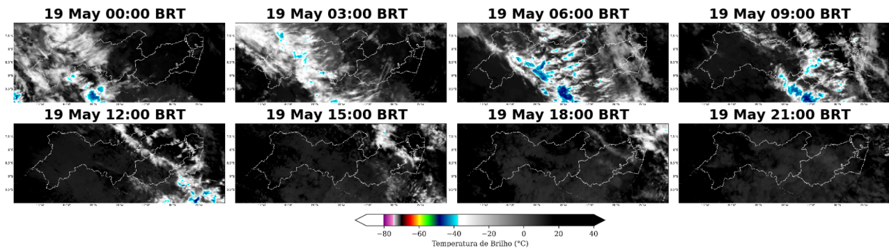
Figura 2: Imagens realçadas do satélite GOES-16 das 00 BRT até 21 BRT (a cada 3 horas) para o dia 19 de maio.
