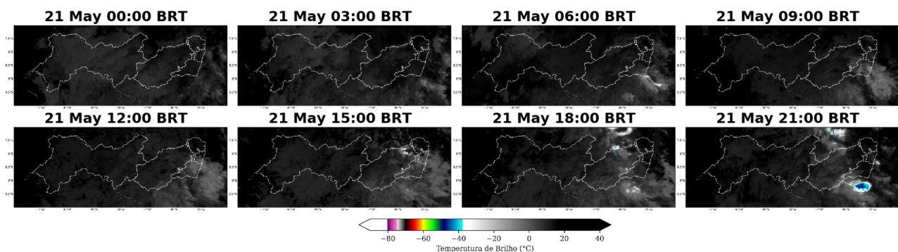
Figura 4: Imagens realçadas do satélite GOES-16 das 00 BRT até 21 BRT (a cada 3 horas) para o dia 21 de maio.
