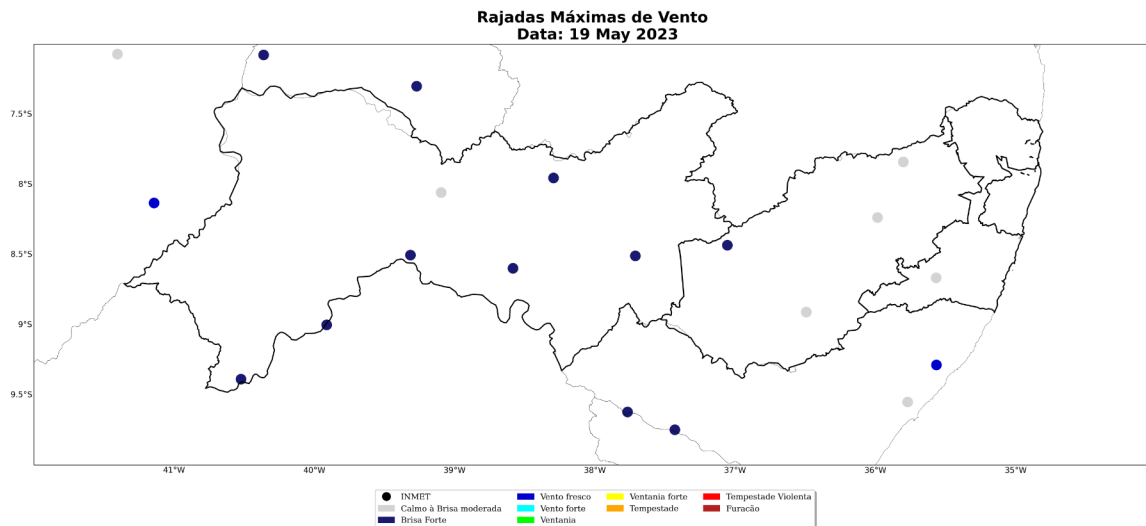
Figura 19: Rajada de vento sobre o estado de Pernambuco para o dia 19 de maio, baseado nas estações meteorológicas do INMET
