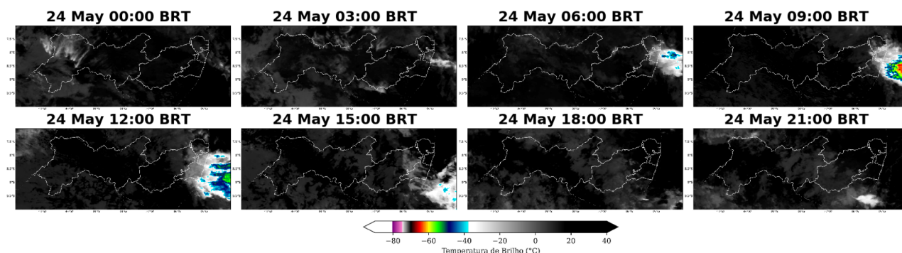
Figura 7: Imagens realçadas do satélite GOES-16 das 00 BRT até 21 BRT (a cada 3 horas) para o dia 23 de maio.
